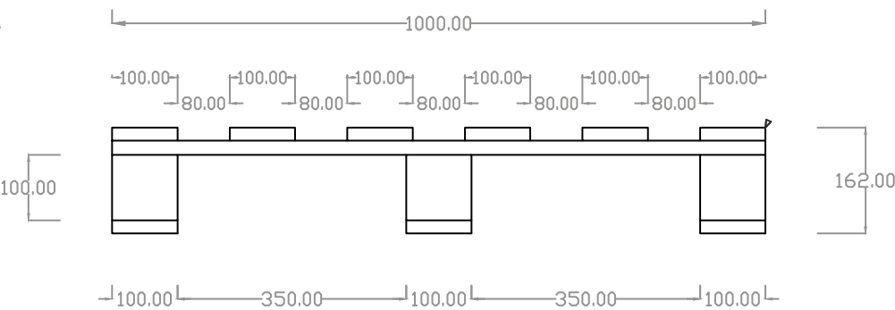
VISTA LATERAL
