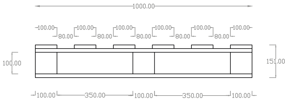
VISTA LATERAL
