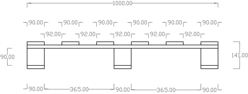
VISTA LATERAL
