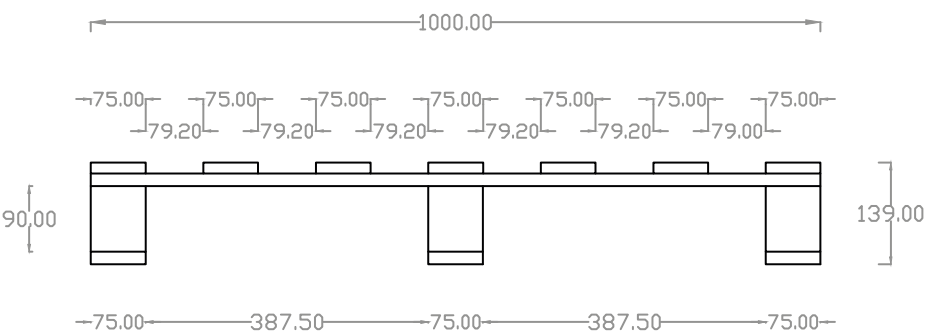
VISTA LATERAL
