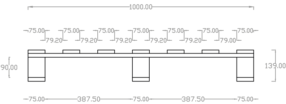
VISTA LATERAL
