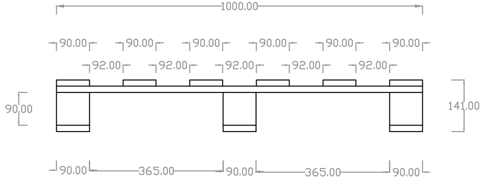
VISTA LATERAL
